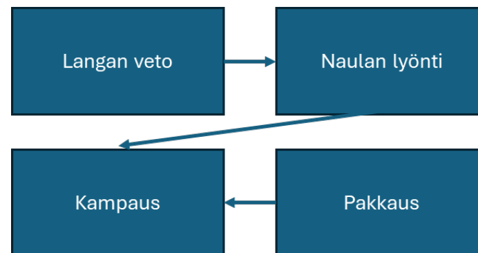
Kuva 2. Tuotteiden valmistusprosessi
